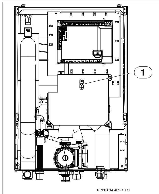
Afb. 6 Binneneenheid AWES
